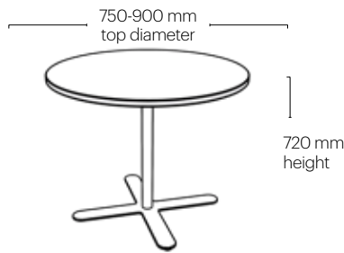
Bud Round Table 720h BUD-RD-750-900
