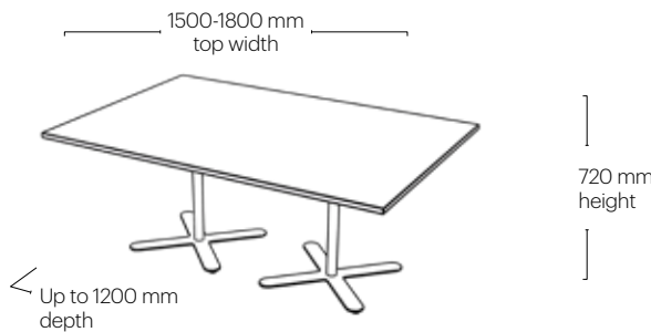
Bud Rectangular Table 720h BUD-720H-REC12-15-18
